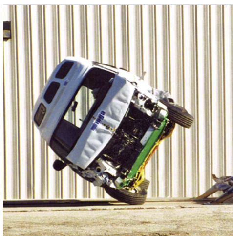
Les essais dynamiques de capotage ont pour objectif de réduire le nombre de blessures et de morts qui surviennent lorsque les occupants sont éjectés au cours d'un capotage.
