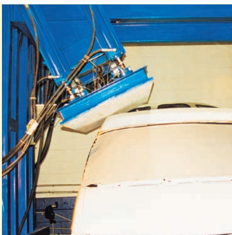
Les essais de résistance à l'écrasement du toit visent à réduire le nombre de morts et de blessures qui surviennent à la suite de l'écrasement du toit au cours d'un capotage.
