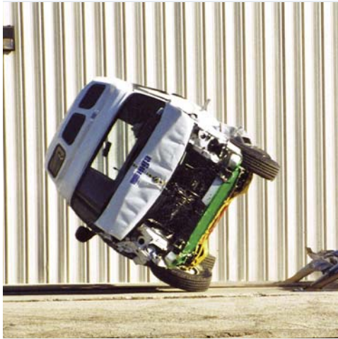
Les essais dynamiques de capotage visent à réduire le nombre de morts et de blessures qui surviennent à la suite de l'éjection des occupants au cours d'un capotage.
