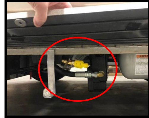
36.6 Raccord externe de barbecue
