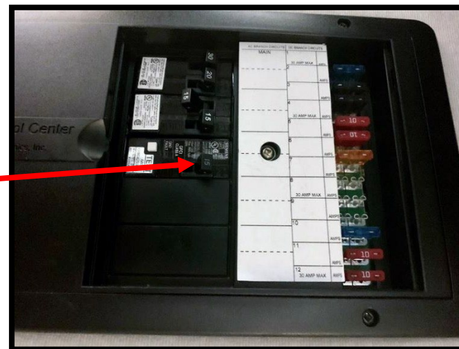
Panneau de disjoncteurs et de fusibles au-dessus du siège du conducteur
