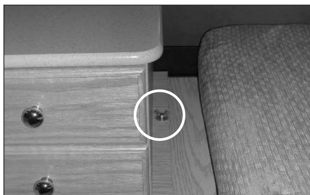
Photo B-P7: Écrou à oreilles retenant la table de chevet; on y accède sur les côtés (Popular).
