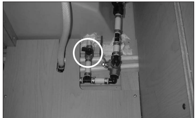
Photo G-P7: Robinet de vidange du réservoir intérieur en position fermée
